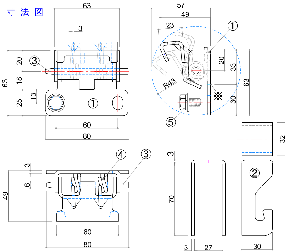
寸法図
