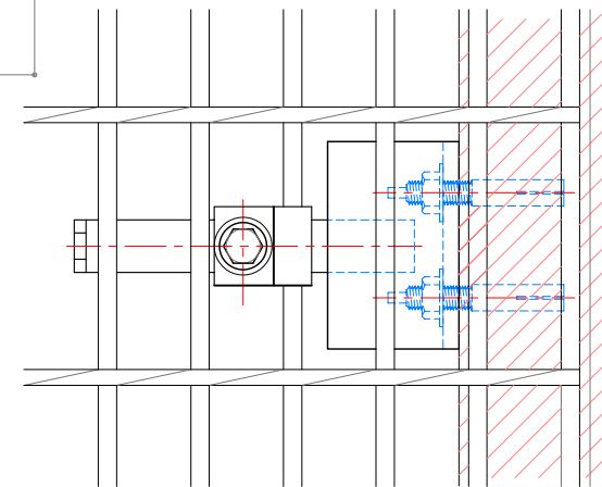
平面図
