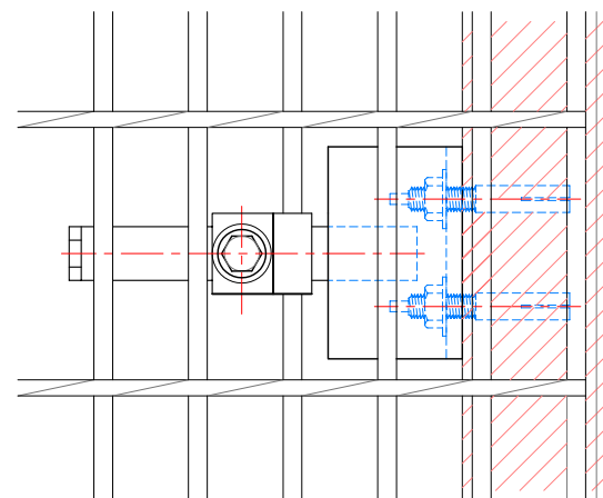
ブラケット取付け壁面に平行なベアリングバーに設置する場合
