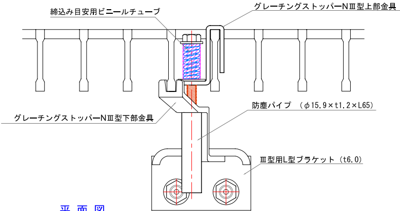
平面図
